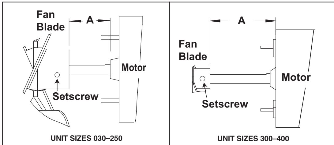
Figure 3. Fan Spacing
