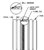
12"-60" (300-1500mm) N-12 WT IB
