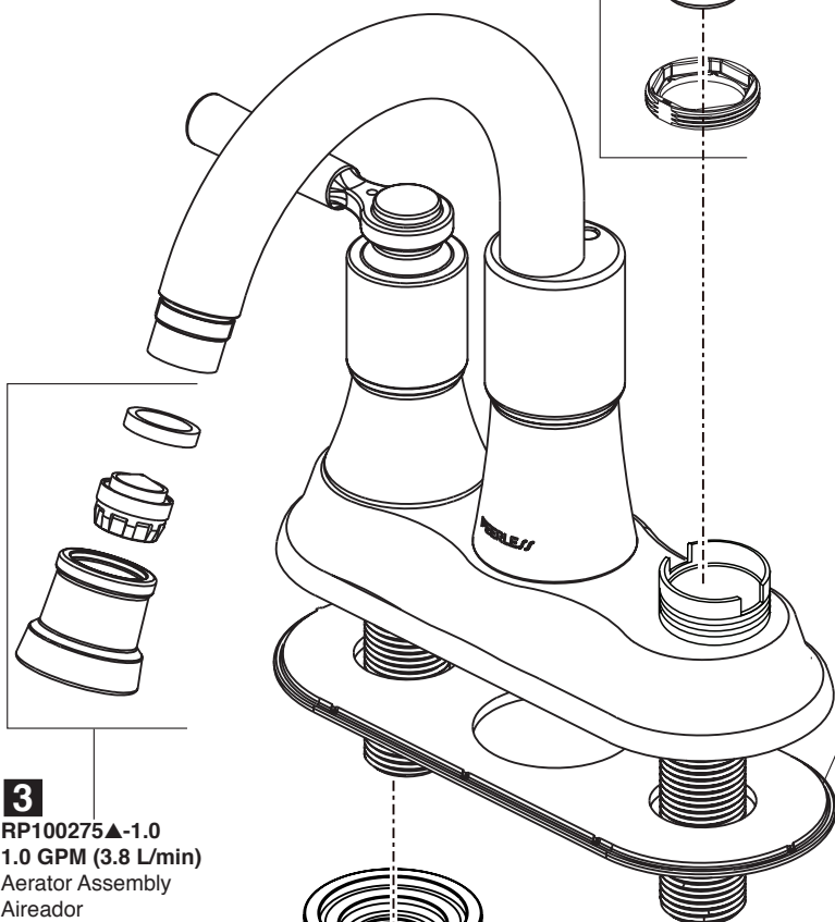
RP5412 Locknuts Contratuercas Écrous de Blocage
